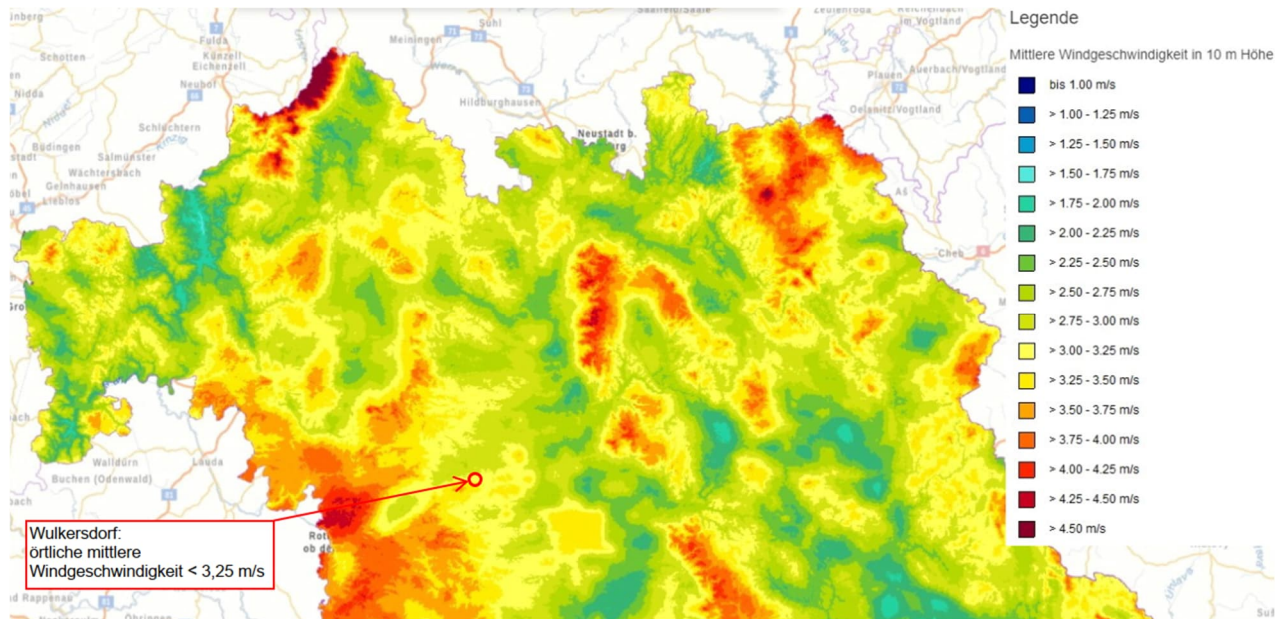
Abb. 2: Ausschnitt Bayerischer Windatlas mit Lage der Maßnahme
